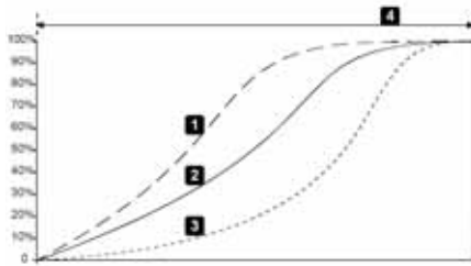
Профили ААС
