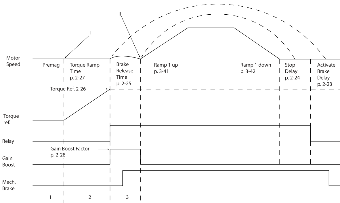
Рисунок 3.5 Последовательность отпущения тормоза при управлении механическим тормозом подъемного механизма
